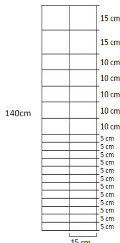
Stålstängsel 140cm/20/15
