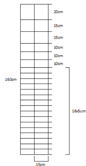
Stålstängsel 160cm/23/15
