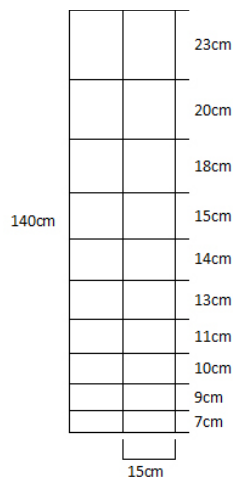
Stålstängsel 140cm/11/15
